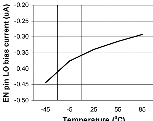
EN Pin LO Bias Current vs. Temp.
