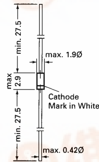
Glass case JEDEC DO-34
