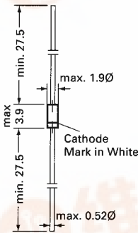
Glass case JEDEC DO-35
