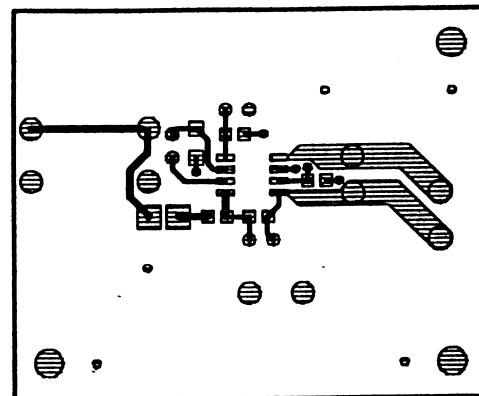
Top Layer
