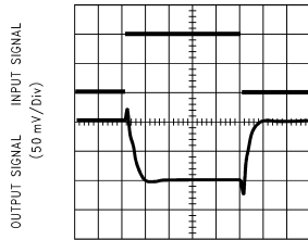
TIME (10 \mu s /Div) DS011422-30
