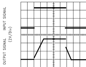
TIME (100 \mu s /Div) DS011422-33
