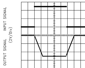
TIME (100 \mu s /Div) DS011422-31
