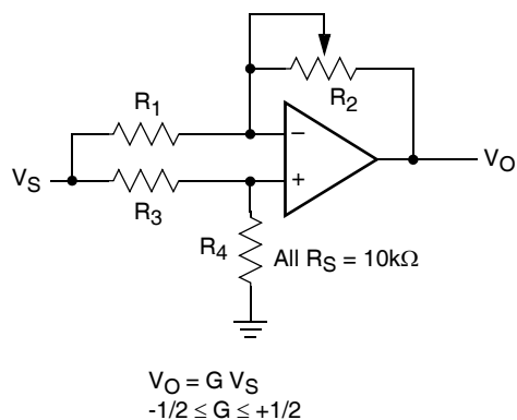
Attenuator
