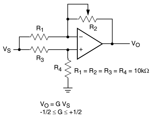
Attenuator
