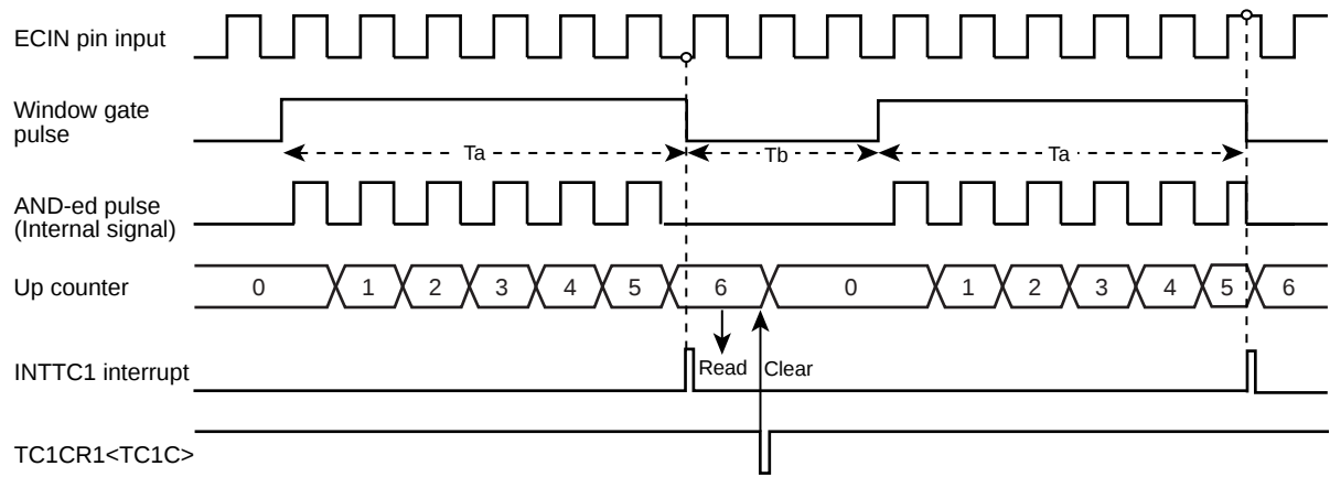
a) TC1CR2<SEG> = '0'
