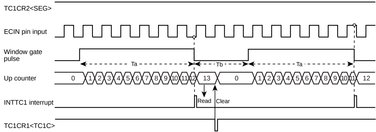
a) TC1CR2<SEG> = '1'
