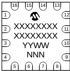
16-Lead QFN*
