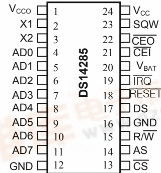
DIP/SO
