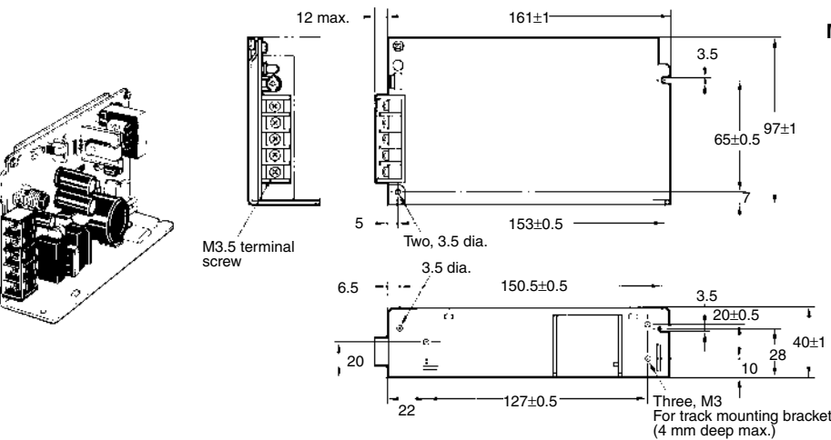
S82J-050 □□□ (50 W)
