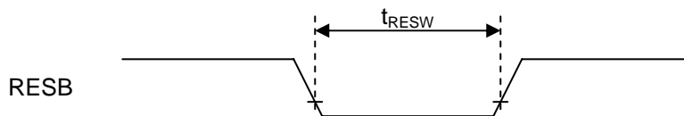
【Fig 7-3 Reset Timing Signal】
