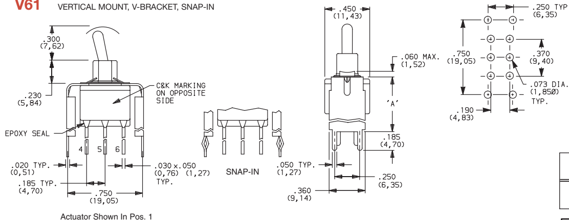
E201MD1_BE DPDT
