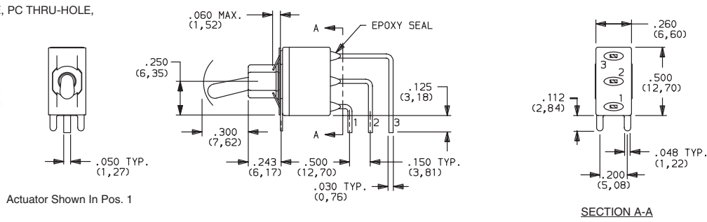
E101MD1AV2BE
