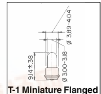
T-1 Miniature Flanged
