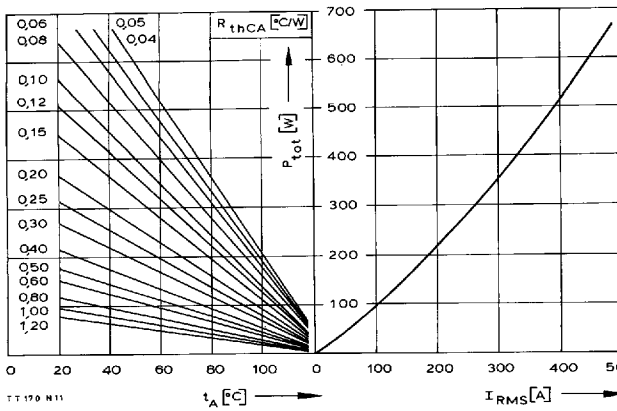
Bild/Fig. 7 W1C – Einphasen-Wechselwertschaltung/Single-phase inverse parallel circuit Höchstzulässiger Strom I_{RMS} in Abhängigkeit von der Umgebungstemperatur t_A . Maximum allowable current I_{RMS} versus ambient temperature t_A . Parameter: Wärmewiderstand zwischen Powerblock und Umgebung/ thermal resistance case to ambient R_{thCA}
