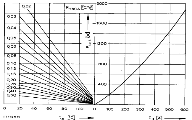
Bild/ Fig. 6 B6 – Sechspuls-Brückenschaltung/Six-pulse bridge circuit Höchstzulässiger Ausgangsstrom I_d in Abhängigkeit von der Umgebungstemperatur t_A . Maximum allowable output current I_d versus ambient temperature t_A . Parameter: Wärmewiderstand zwischen Powerblock und Umgebung/ thermal resistance case to ambient R_{thCA}
