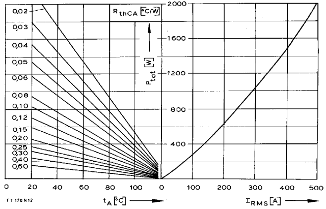
Bild/Fig. 8 W3C – Dreiphasen-Wechselwertschaltung/Three-phase inverse parallel circuit Höchstzulässiger Strom je Phase I_{RMS} in Abhängigkeit von der Umgebungstemperatur t_A . Maximum allowable current per phase I_{RMS} versus ambient temperature t_A . Parameter: Wärmewiderstand zwischen Powerblock und Umgebung/ thermal resistance case to ambient R_{thCA}
