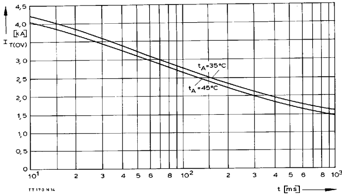
Bild/Fig. 9 Grenzstrom je Zweig I_{T(OV)M} bei Luftselbstkühlung, t_A = 45^\circ\text{C} und verstärkter Luftkühlung, t_A = 35^\circ\text{C} , Kühlkörper KP0,33S, V_{RM} = 0,8 V_{RRM} . Limiting overload on-state current per arm I_{T(OV)M} at natural ( t_A = 45^\circ\text{C} ) and forced ( t_A = 35^\circ\text{C} ) cooling, heatsink type KP0,33S, V_{RM} = 0,8 V_{RRM} . a – Belastung nach Leerlauf/current surge under no-load conditions b – Belastung nach Betrieb mit Dauergrenzstrom I_{TAVM} Current surge occurs during operation at limiting mean on-state current rating I_{TAVM}
