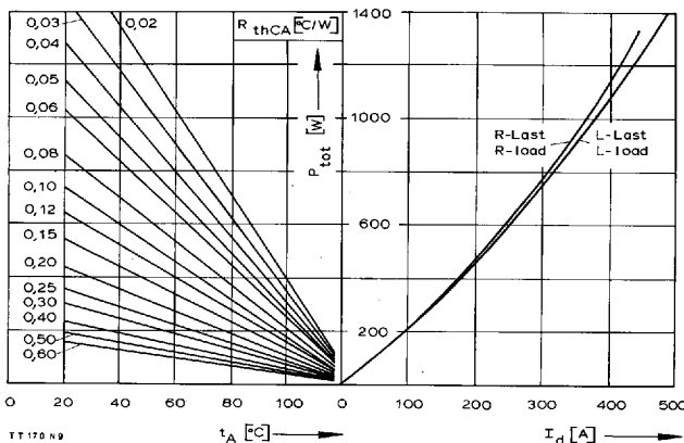
Bild/ Fig. 5 B2 – Zweipuls-Brückenschaltung/Two-pulse bridge circuit Höchstzulässiger Ausgangsstrom I_d in Abhängigkeit von der Umgebungstemperatur t_A . Maximum allowable output current I_d versus ambient temperature t_A . Parameter: Wärmewiderstand zwischen Powerblock und Umgebung/ thermal resistance case to ambient R_{thCA}
