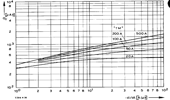
Bild/Fig. 10 Sperrverzögerungsladung Q_R in Abhängigkeit von der abkommütierenden Stromsteilheit -di/dt bei t_{vj} = t_{vj \max} , V_R = 0,5 V_{RRM} , V_{RM} = 0,8 V_{RRM} . Der angegebene Verlauf ist gültig für 90% aller Elemente. Recovered charge versus the rate of decay of the forward on-state current -di/dt at t_{vj} = t_{vj \max} , V_R = 0,5 V_{RRM} , V_{RM} = 0,8 V_{RRM} . These curves are valid for 90% of all devices. Parameter: Durchlaßstrom I_{TM} /On-state current I_{TM}
