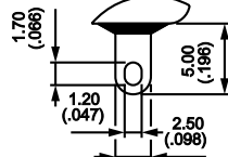
Solder Lug
