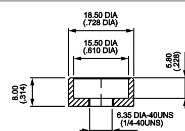
U825 For caps U630 & U3400
