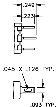
SOLDER LUG
