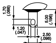
Solder lug
