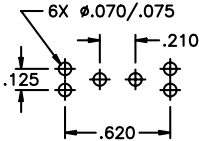
P.C. LAYOUT
