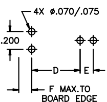
P.C. LAYOUT
