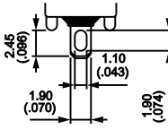
S0 Solder lug
