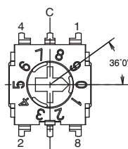
RTE10 10 POSITION
