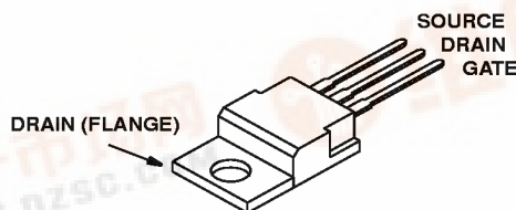
JEDEC TO-220AB
