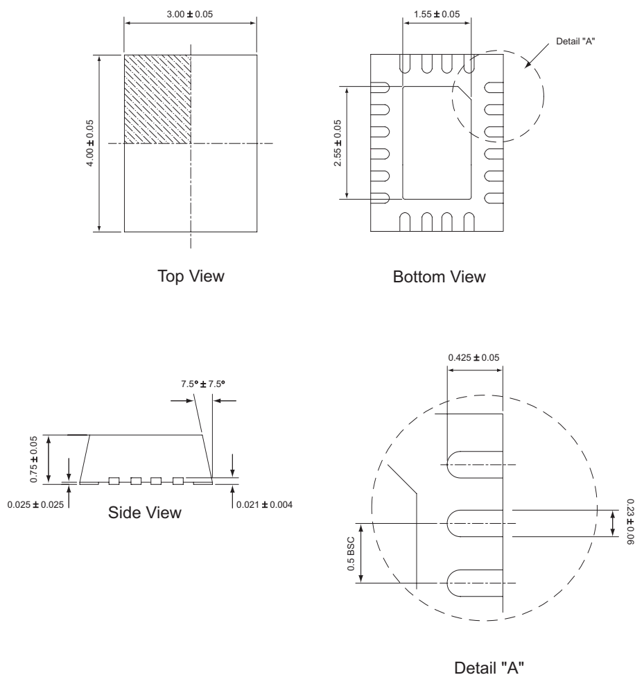
TQFN34-20
