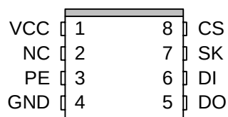
8pin SON
