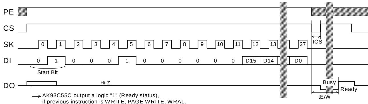
WRAL (AK93C55C)
