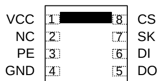
8pin USON
