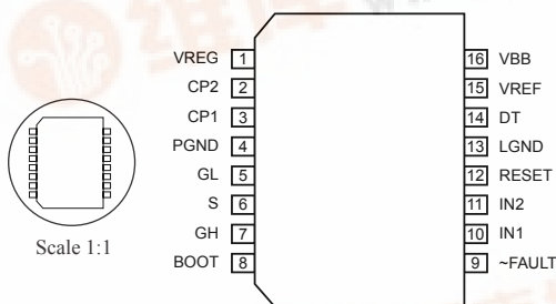
A3946KLB SOIC
