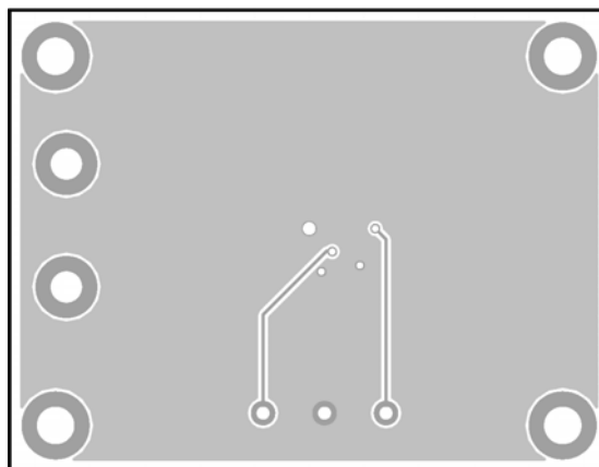
Figure 3—Bottom Layer
