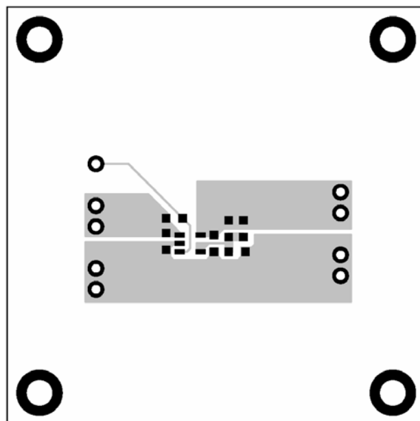
Figure 2—Top Layer
