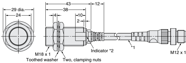
E2EQ-X8X1-M1J
