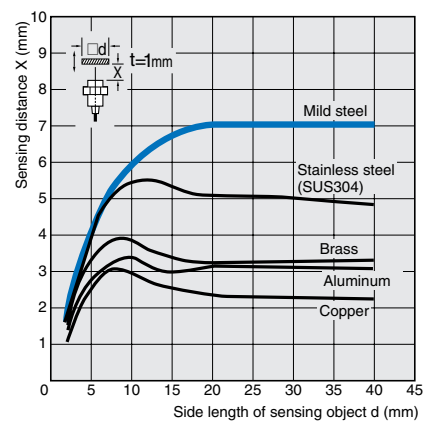
E2EQ-X7D1(-M1GJ)
