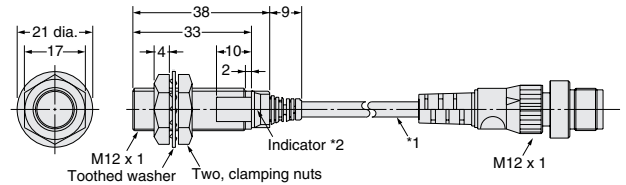
E2EQ-X4X1-M1J
