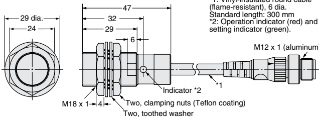
E2EQ-X7D1-M1GJ
