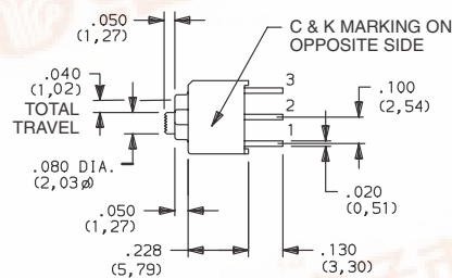
Actuator Shown In Pos. 1
