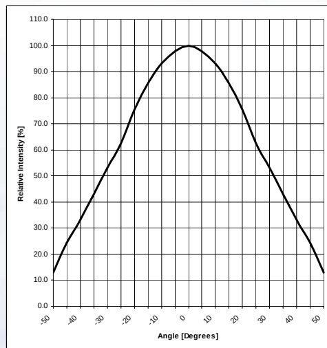
Radiation Pattern (orthogonal) (CW)
