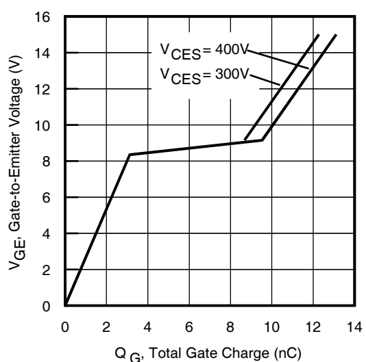
Fig. 24- Typ. V_{GE} vs. Q_G
