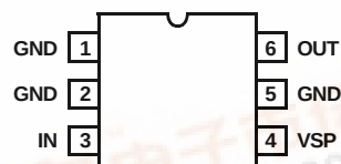
6 LD SC-70
