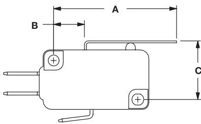
FIG. 3 Lever
