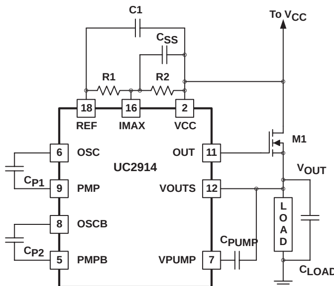
Figure 5. MOSFET Softstart Diagram
