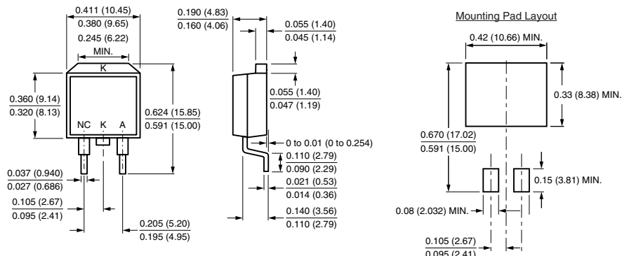
TO-263AB
