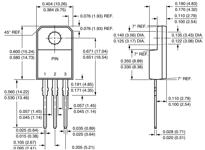
ITO-220AB
