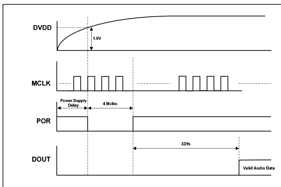
Figure 7 POR Timing
