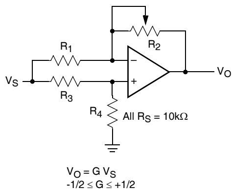
ATTENUATOR
