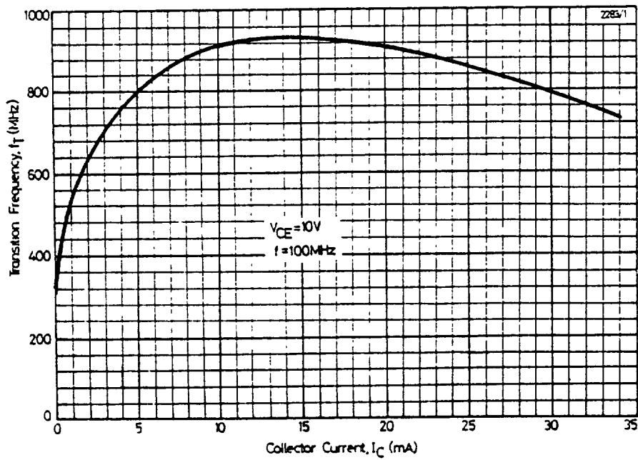
I_C/f_T (ZTX312)
