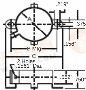
VR1, 3 & 4
