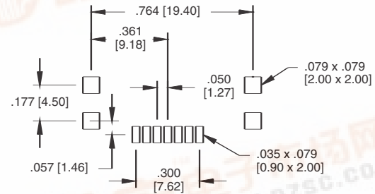
SATA-B-PL-SMT-K
