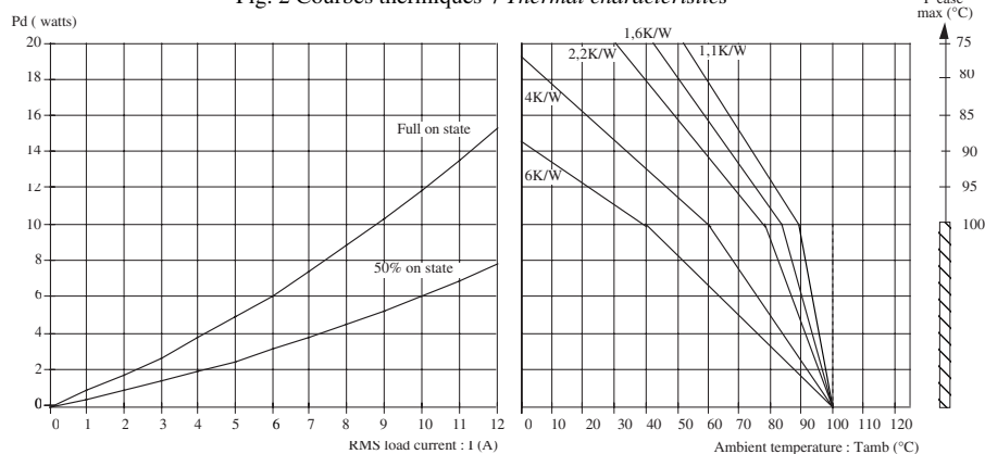
Fig. 2 Courbes thermiques / Thermal characteristics
