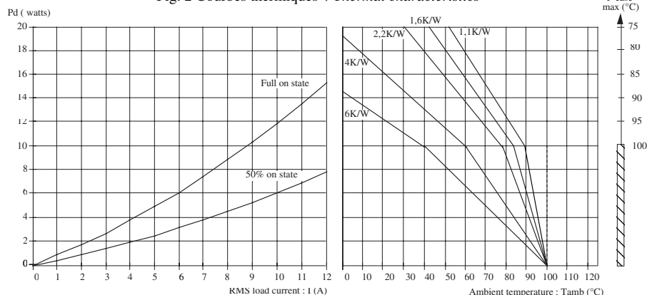
Fig. 2 Courbes thermiques / Thermal characteristics
