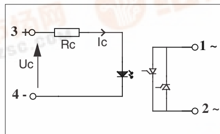
Caractéristiques de commande (à 20°C) / Control characteristics (at 20°C)
