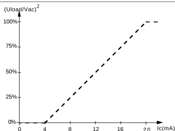
Fig.3 Caractéristique de transfert, linéarisé en U^2 Transfer characteristic with U^2 linearisation.
