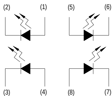
Polarity
