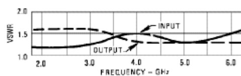
VSWR
