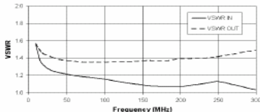
VSWR
