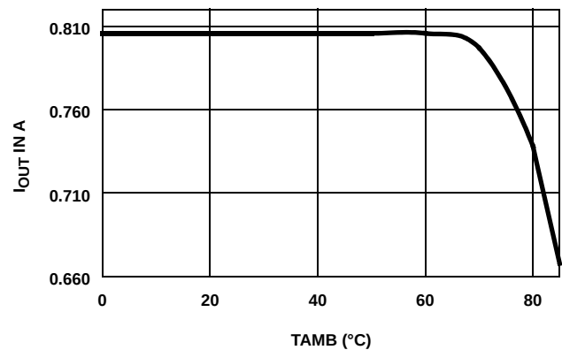
FIGURE 3. OUTPUT CURRENT DERATING 40 LD 6x6 QFN: I OUT_max vs T AMB
