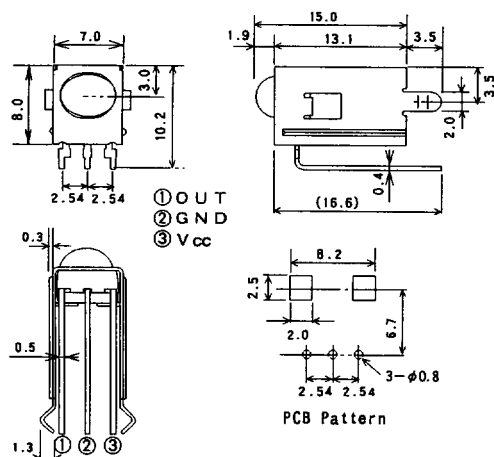
NJL64H000 UNIT : mm
