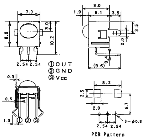
NJL62H000 UNIT : mm
