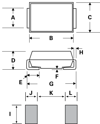
DO-214AC (SMA)
