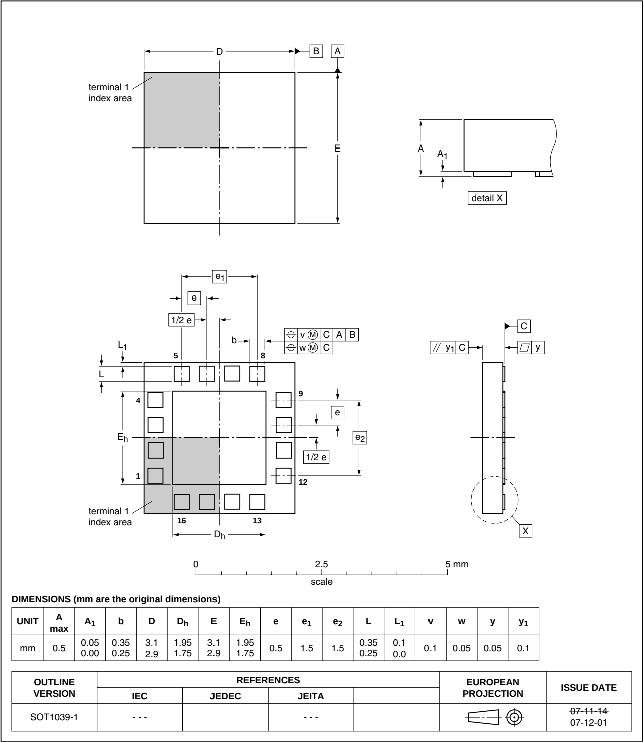
Fig 25. Package outline SOT1039-1 (HXQFN16U)
