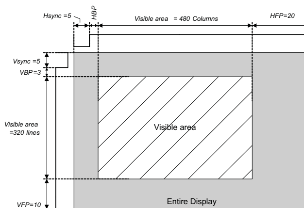
Figure 29. HVGA Display
