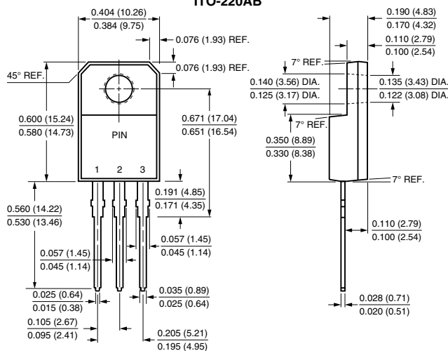
ITO-220AB
